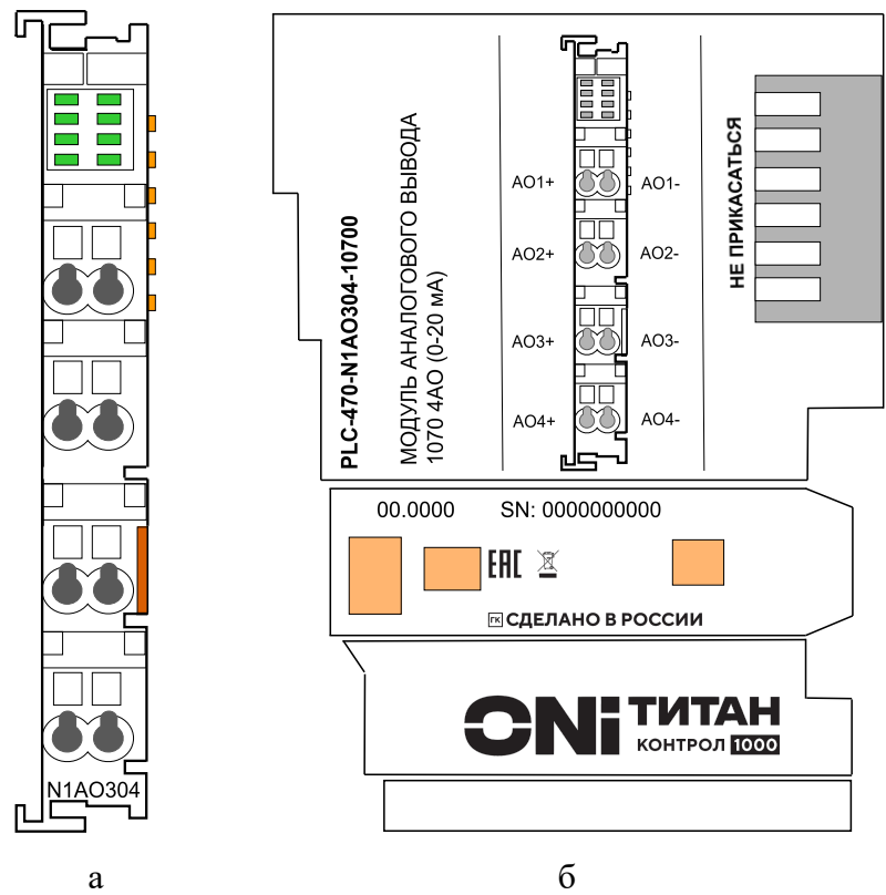
Рисунок 1 – Модуль N1AO304 (а – вид спереди, б – вид справа)
