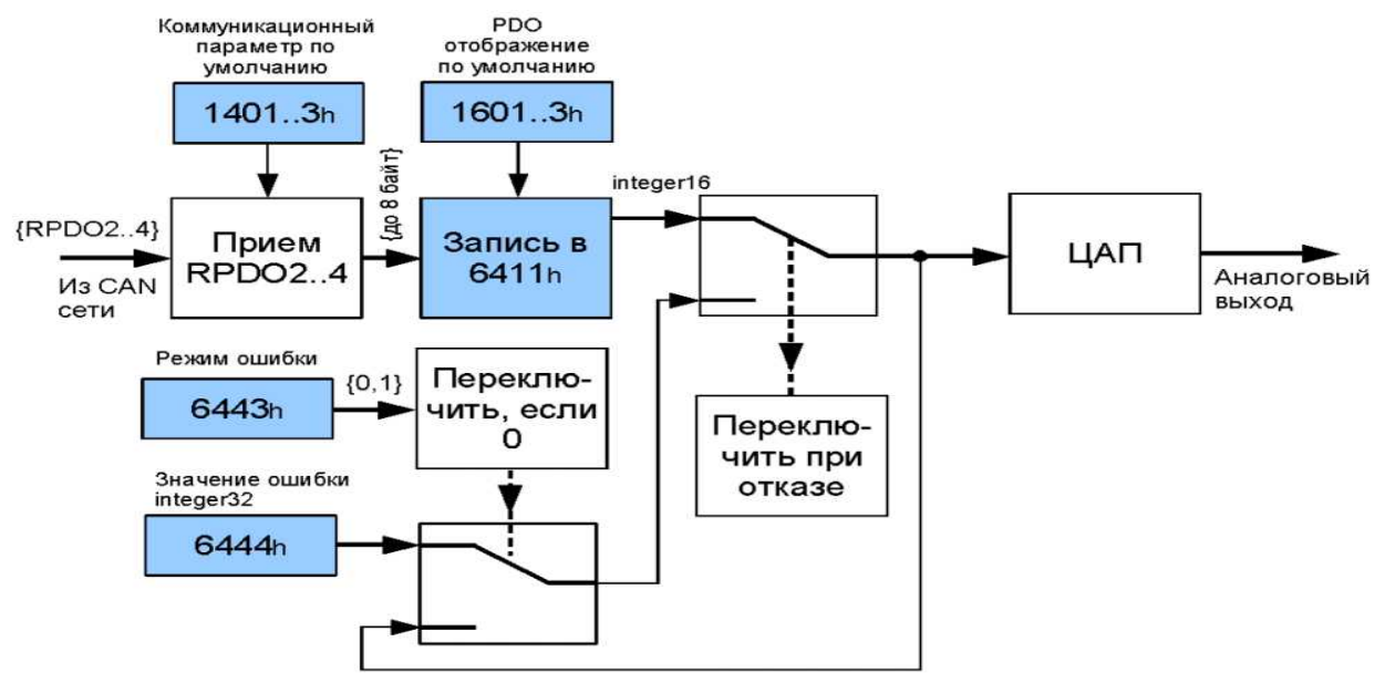
Рисунок 2 – Алгоритм работы модуля аналогового вывода
