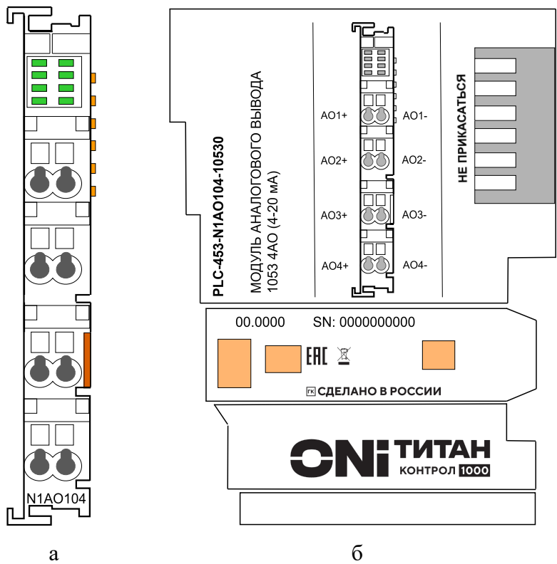
Рисунок 1 – Модуль N1AO104 (а – вид спереди, б – вид справа)
